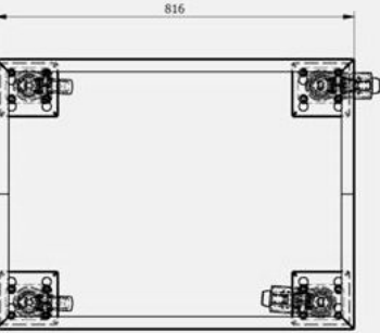
Gesamtlänge Wagen
