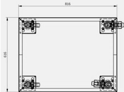
Gesamtlänge Wagen
